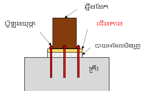
វិធីសាស្ត្រចាប់ភ្ជាប់ឆ្អឹងដែកដោយជើងតាង
